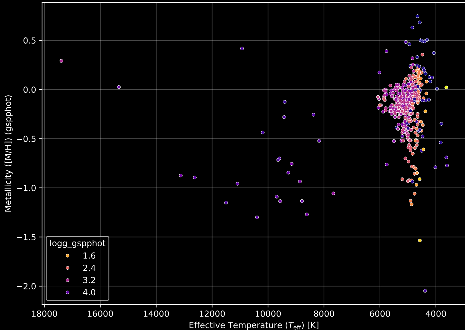
APOGEE DR17 Field: [210-08] Stellar Population Parameters (n= 478)
